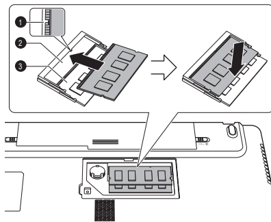
Abbildung 3-12 Speichermodul einsetzen (L770/L775/L770D/L775D)
