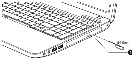
Abbildung 3-7 Lade manuell öffnen (L770/L775/L770D/L775D)
