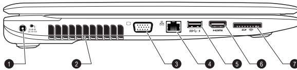
Abbildung 2-8 Linke Seite des Computers
