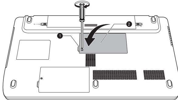
Abbildung 3-13 Speichermodulabdeckung einsetzen (L770/L775/L770D/L775D)
