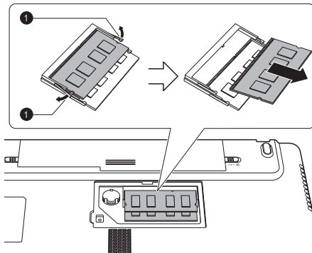
Abbildung 3-14 Speichermodul entfernen (L770/L775/L770D/L775D)
